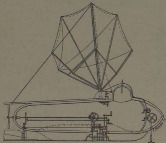
ROBERT FULTON, américain, construit en France. — 1797.
