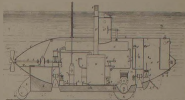
LAKE, américain. — 1896.
