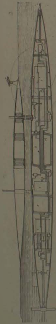
Haight et Wood. — 1886. Sous-marin à flotteur : longueur, 25 mètres ; diamètre, 1 m. 75 ; propulsion par hélice et moteur à acide carbonique liquide ; immersion par introduction d'eau ; armé de torpilles.
