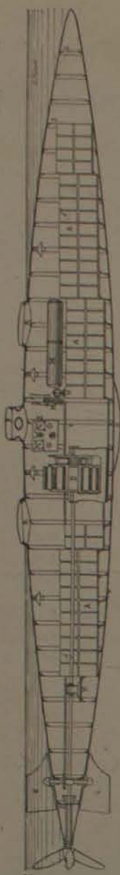
GUSTAVE-ZÉDÉ, n° 1, français. — 1888. Gymnote : longueur, 17 m. 30 ; diamètre, 1 m. 80 ; déplacement, 30 tonneaux ; propulsion par l'électricité ; immersion par introduction d'eau, plongée par gouvernail horizontal ; construit en acier.
