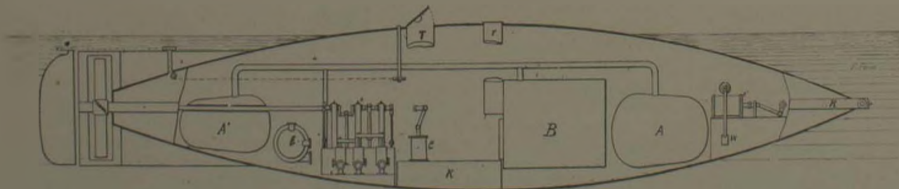
NORDENFELT, suédois. — 1885.
