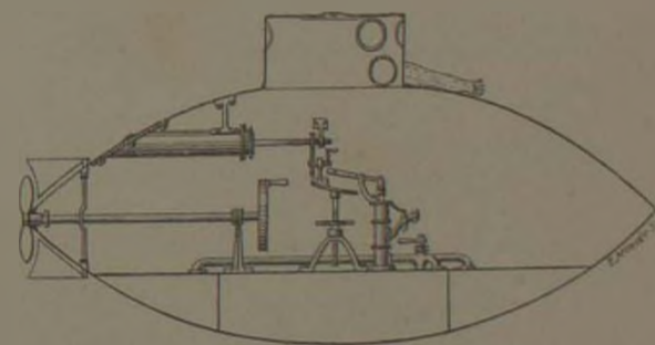
GARRETT. — 1875.
