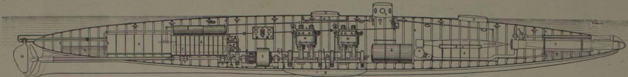
FOREST, français. — 1891.
