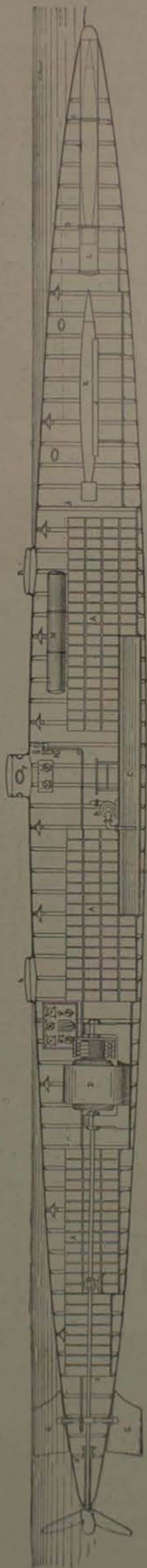
BARON, français. — 1886. Projet de sous-marin à propulsion mixte ; longueur indéterminée ; diamètre, 3 mètres ; propulsion par moteur à pétrole en émergence et par air comprimé en immersion ; mode d'immersion indéterminé. A, moteur à air comprimé ; B, moteur à pétrole ; M, levier de transmission ; R, arbre de couche ; V, volant.
