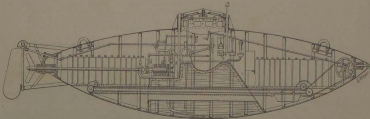
DRZEWIECKI, n° 2, russe. — 1879
