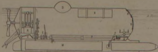
FLAIS, français. — 1885.
