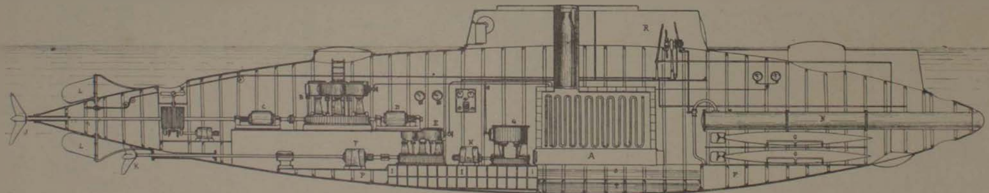
HOLLAND, N° 2, américain. — 1892.
