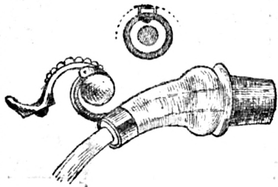
Le bouchon ouvert. — Vue de l'extrémité supérieure
