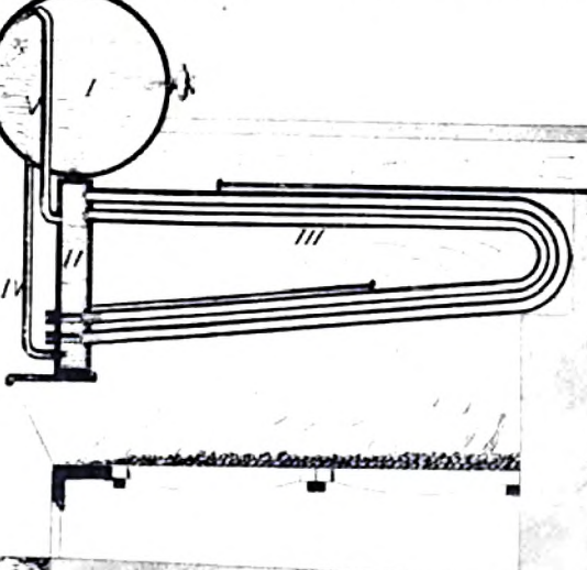
Fig. 2. — I. — Ballon réservoir d'eau et épurateur, dans lequel se fait l'alimentation et où se déposent les dépôts calcaires que l'eau renferme.
