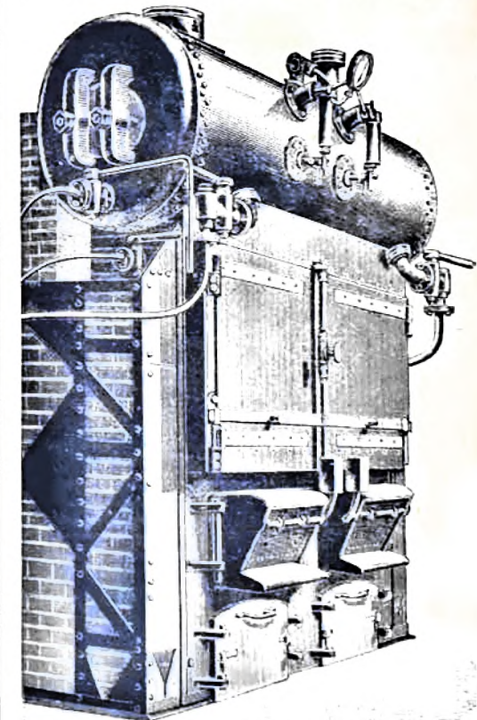
Fig. 3. — Chaudière Solignac de 200 chevaux installée à la station du Secteur électrique du Nord (faubourg St Denis), à Paris.
