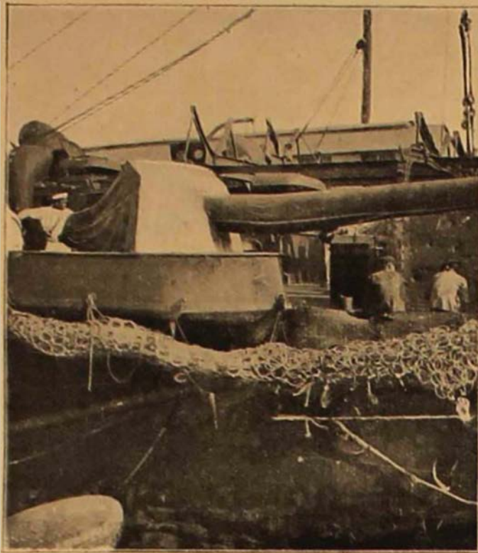
Un des gros canons de tribord de l'Askold tordu par un obus qui a, en outre, tué quatre hommes.
