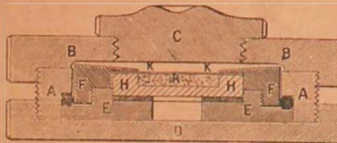
Fig. 1. — Coupe de l'appareil.
