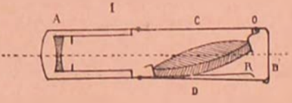
Fig. 2. — Coupe schématique montrant l'intérieur de la jumelle pliée.
