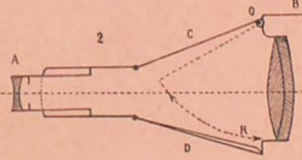
Fig. 3. — Coupe montrant la jumelle ouverte.
